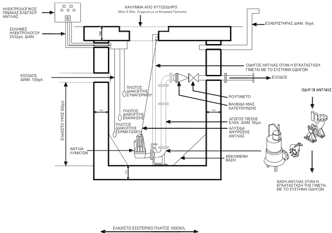
ΤΥΠΙΚΟ ΣΧΕΔΙΟ ΑΝΤΛΙΟΣΤΑΣΙΟΥ ΛΥΜΑΤΩΝ
